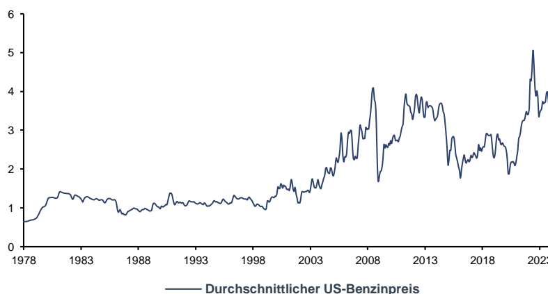
Durchschnittlicher US-Benzinpreis, 01/1978–05/2024
