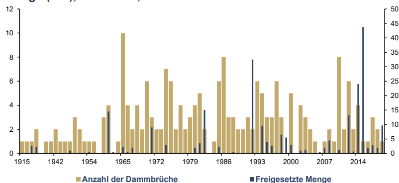
Absetzbecken, Anzahl der Dammbrüche (lhs), und freigesetzte Menge (rhs), in Mio. m 3 , 1915–2019
